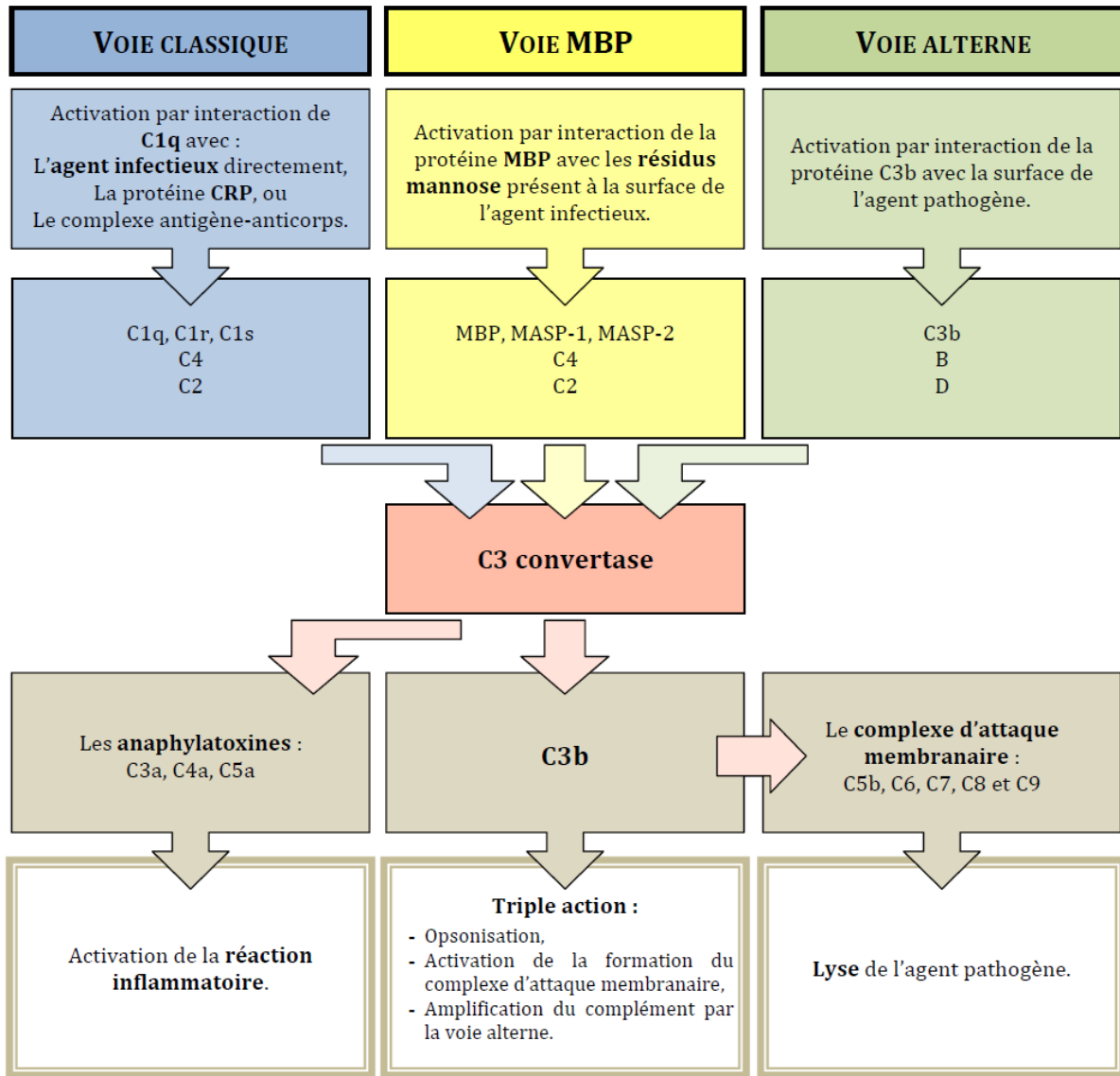
Schéma représentant les grandes étapes et l'action des différentes voies d'activation du complément : la voie classique, la voie MBP et la voie alterne.
